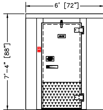
ELEVATION RIGHT HINGE
