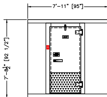
ELEVATION RIGHT HINGE
