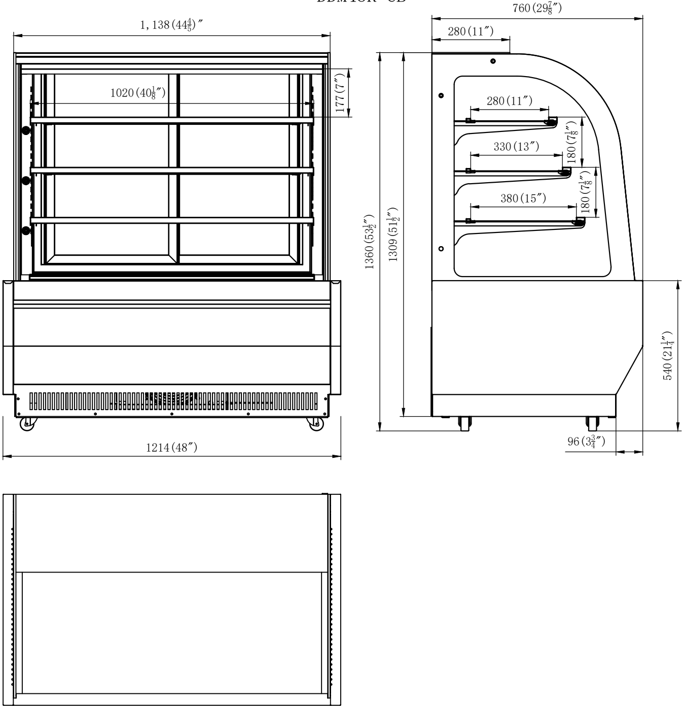
DDM48R-CB
